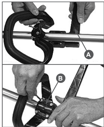
Рис. 4 Установка рабочей рукоятки
