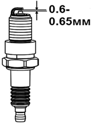
Рис.14 Свеча зажигания
