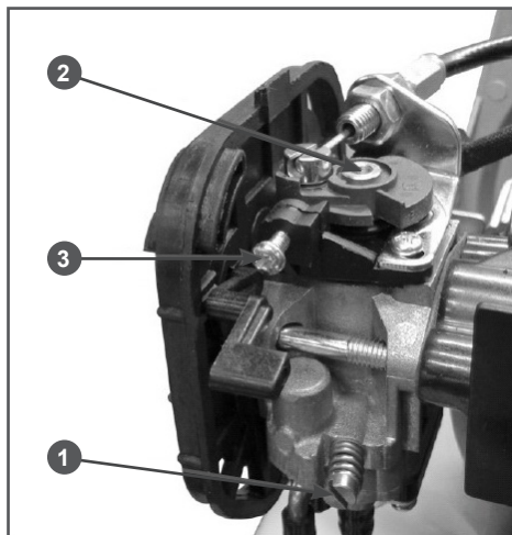
Рис. 15 Расположение винтов карбюратора 1. Винт «L» 2. Винт «H» 3. Винт «T»
