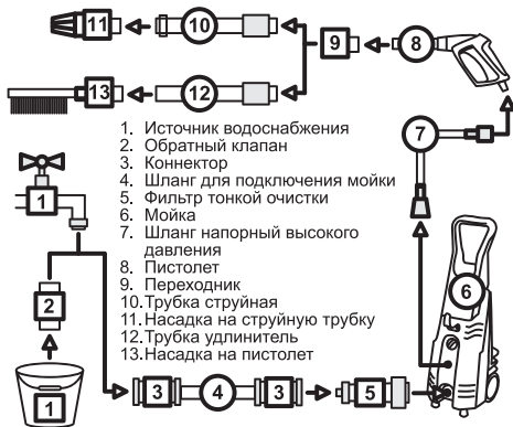
Рис. 12 Схема подключения аппарата мощного высокого давления с дополнительным оборудованием
